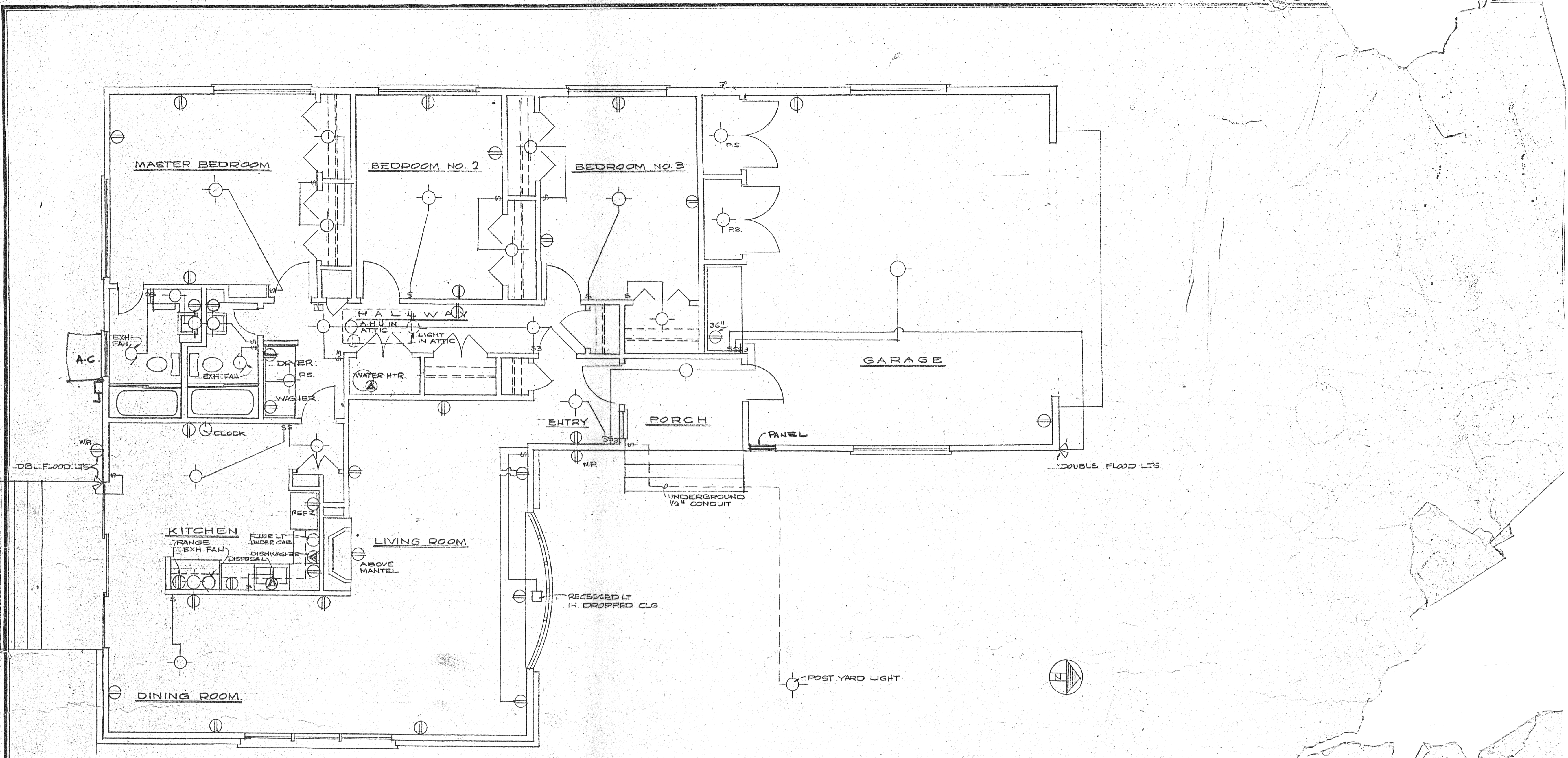
E L E C T R I C A L P L A N 1/4" = 1'-0"
