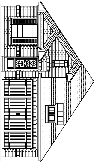
ELEVATION B
