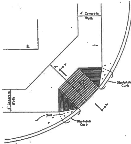
PLAN Scale: 1" = 4'
