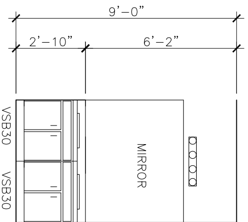
6 M. BATH
