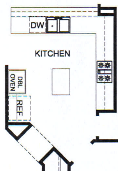
OPTIONAL DOUBLE OVEN
