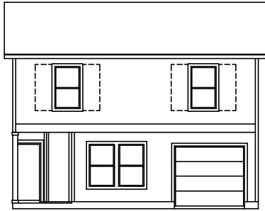
ELEVATION A
