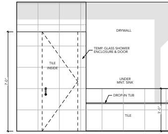
UNIT-E & F BATHROOM-1 SCALE: 1/2" = 1'-0" 12
