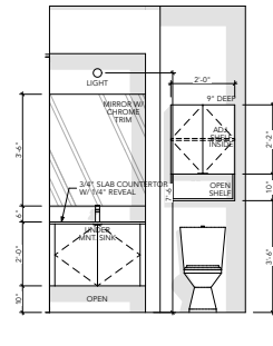
UNIT-F POWDER SCALE: 1/2" = 1'-0" 03
