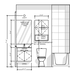
UNIT-F BATHROOM-3 SCALE: 1/2" = 1'-0" 01
