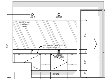
UNIT-E & F BATHROOM-1 SCALE: 1/2" = 1'-0" 11
