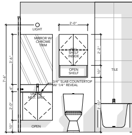
UNIT-E & F BATHROOM-2 SCALE: 1/2" = 1'-0" 13
