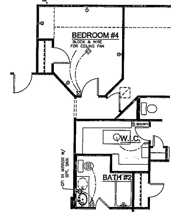
OPT. BEDROOM #4 SCALE: 11x17 1/8" = 1'-0" OPT: BED4 34x22 1/4" = 1'-0"
