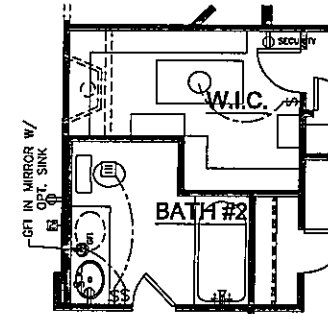
OPT: BATH #2 SCALE: 11x17 1/8" = 1'-0" 34x22 1/4" = 1'-0"
