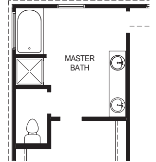
OPTIONAL 60" X 36" TUB & 36" X 36" SHOWER
