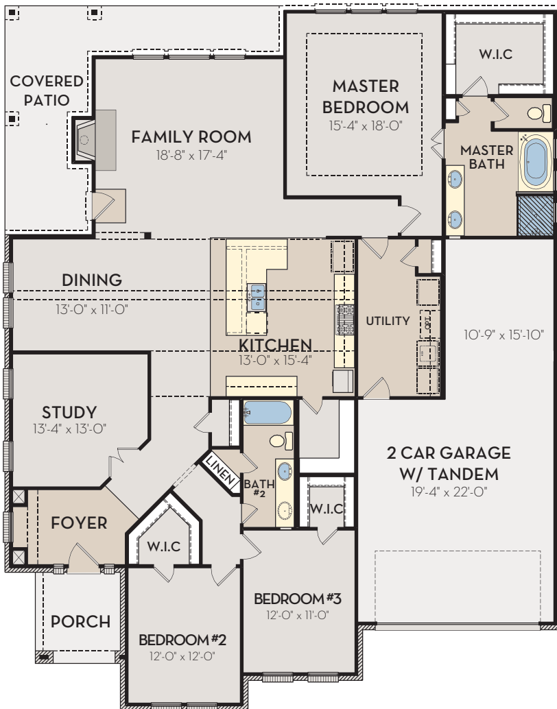
OPT. MASTER DOBLE CLOSET 73 SQ. FT.
