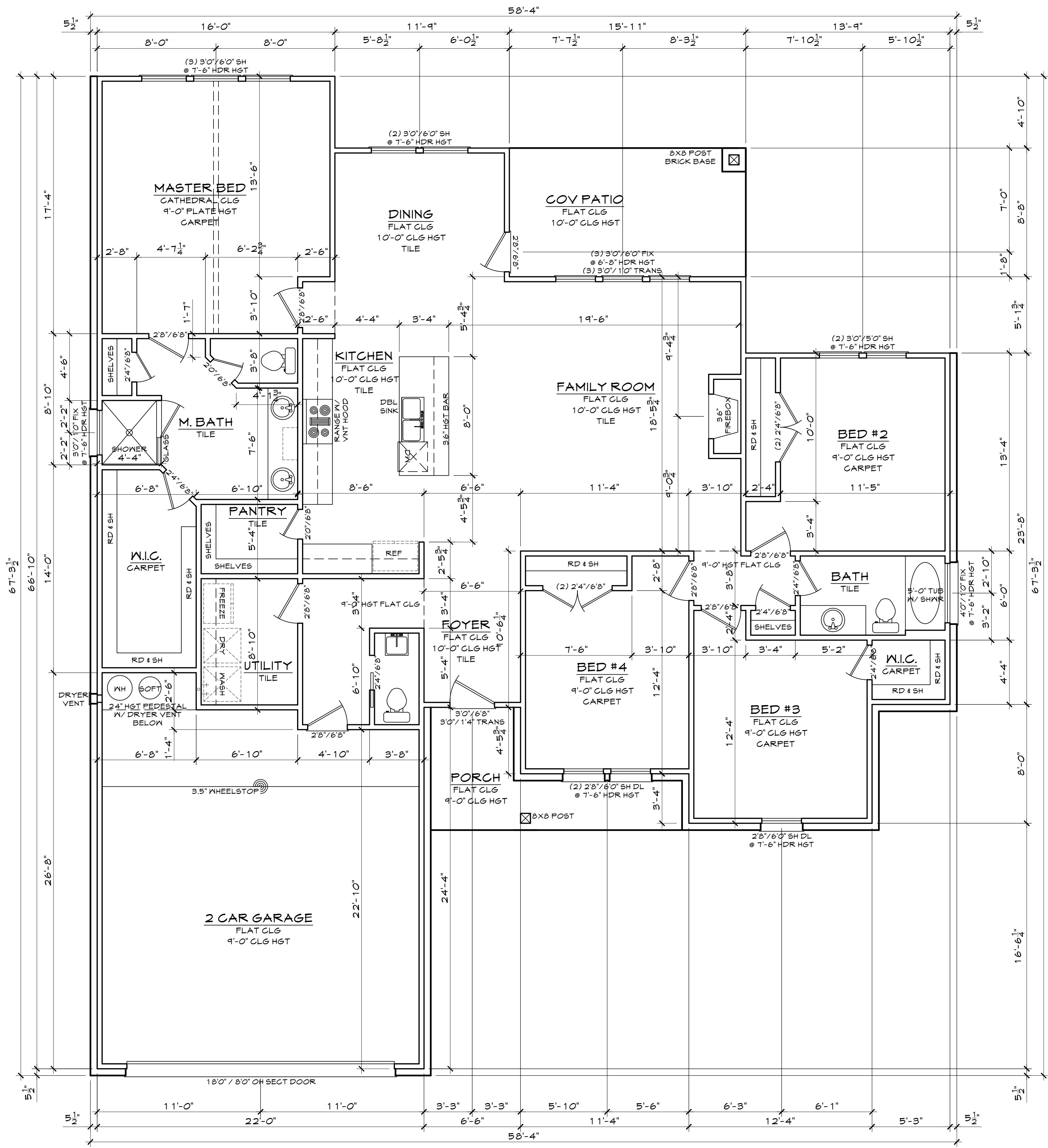
1 FLOOR PLAN A3 SCALE: 1/4" = 1'
