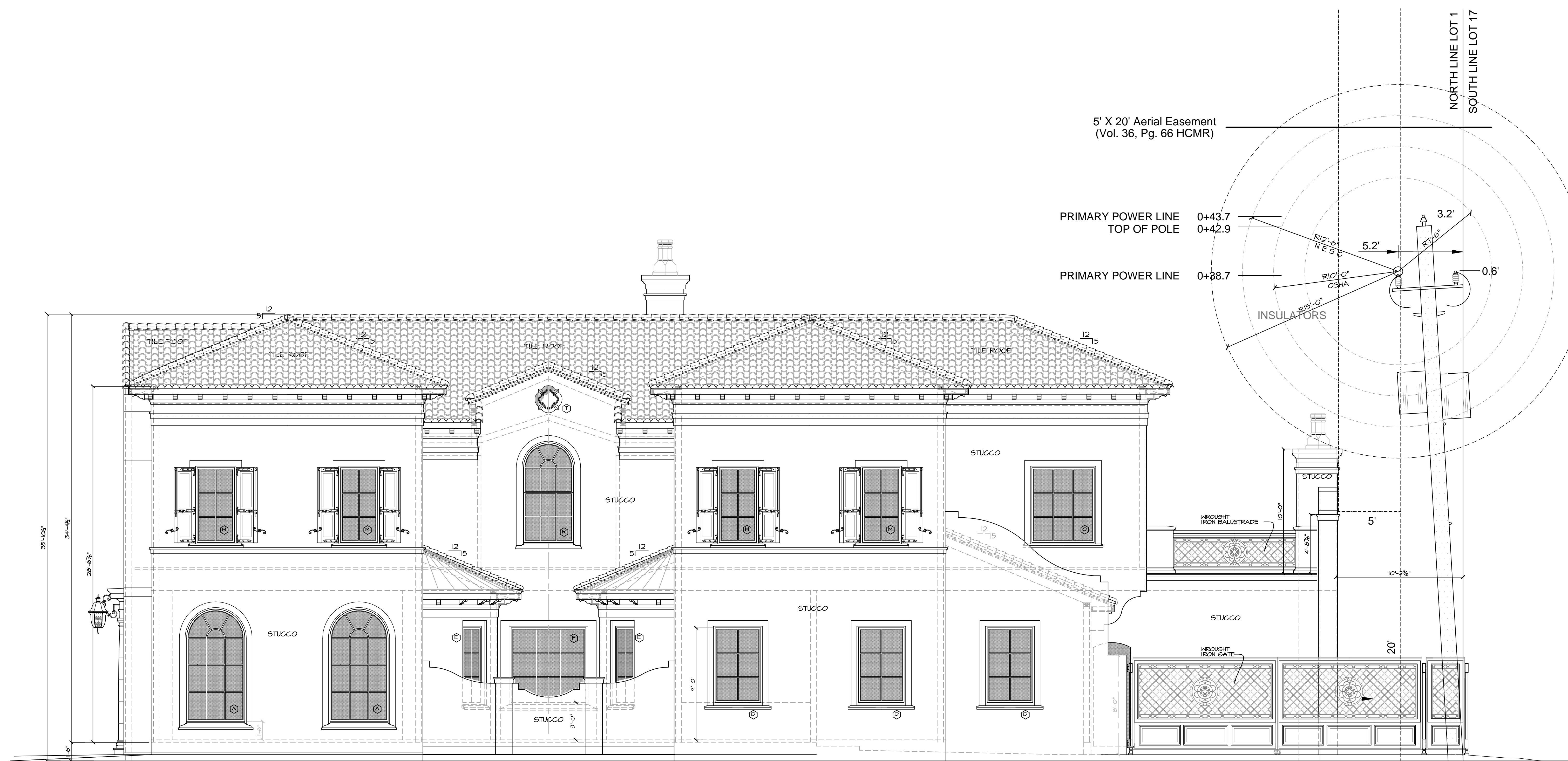
RIGHT ELEVATION
