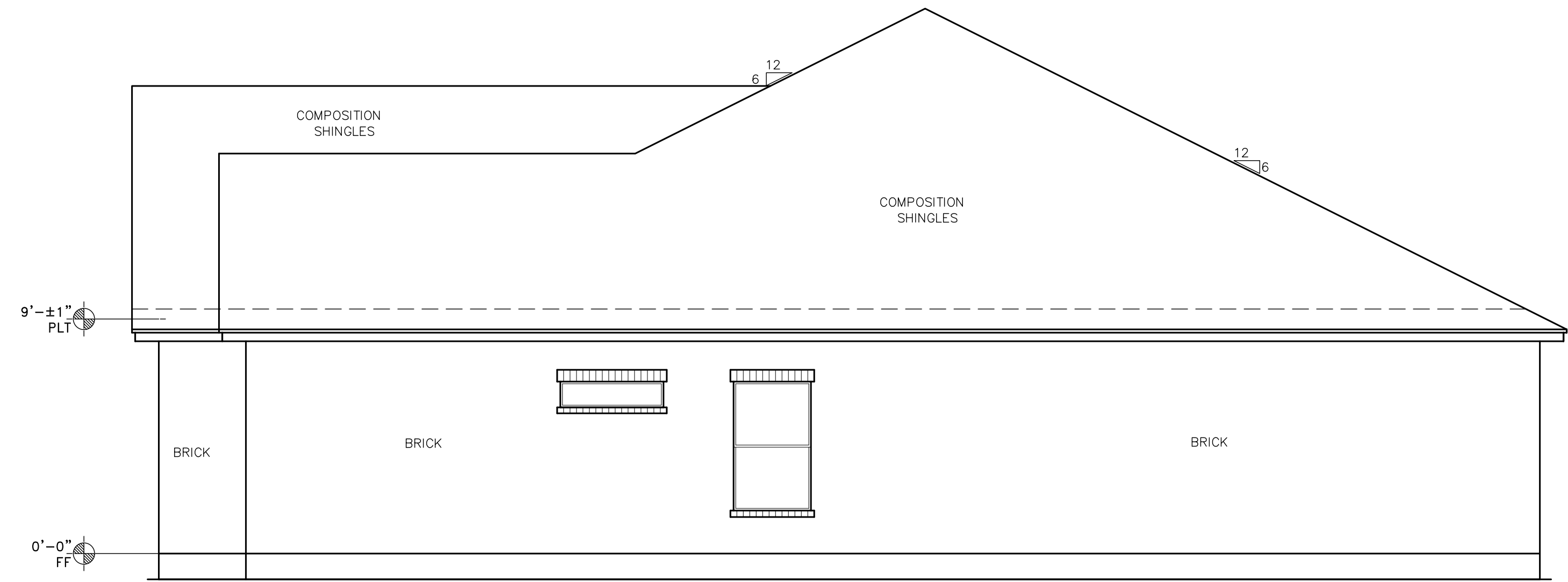
2 RIGHT SIDE VIEW A2 SCALE: 1/4" = 1'
