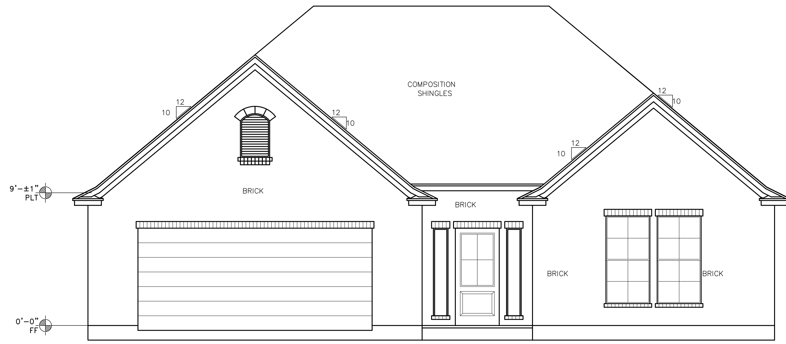
1 FRONT VIEW A1 SCALE: 1/4" = 1'
