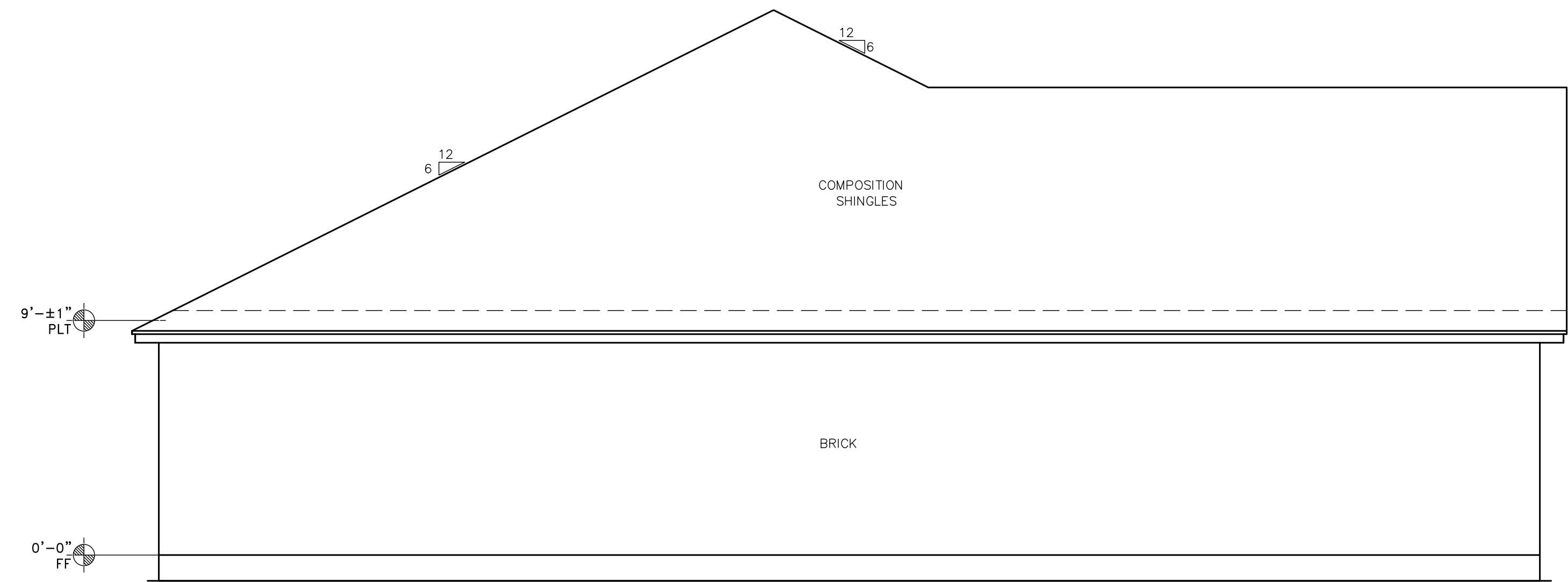
2 LEFT SIDE VIEW A1 SCALE: 1/4" = 1'
