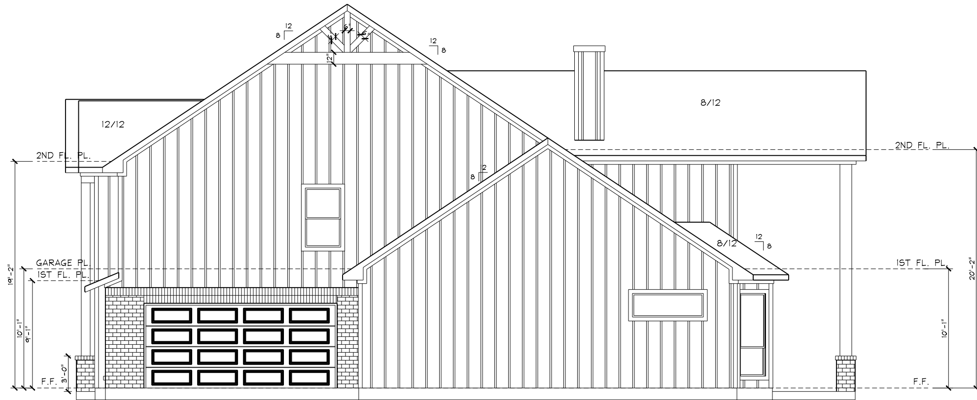
RIGHT ELEVATION
