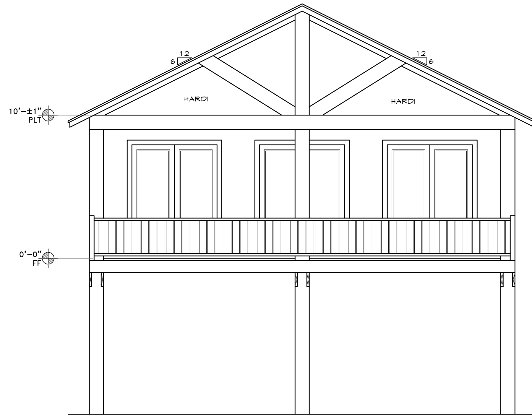
1 FRONT VIEW A1 SCALE: 1/4" = 1'
