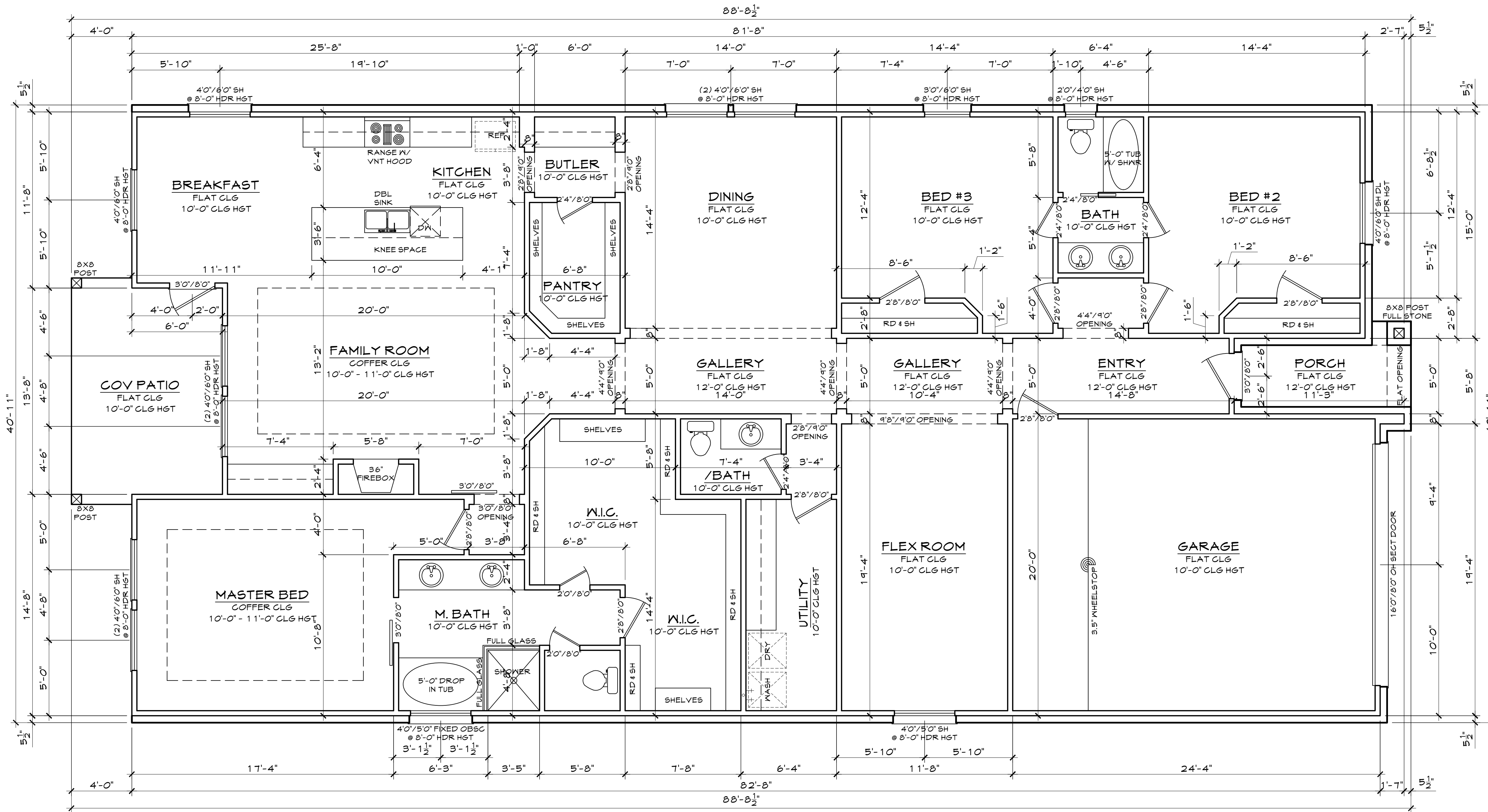
1 FLOOR PLAN A3 SCALE: 1/4" = 1'
