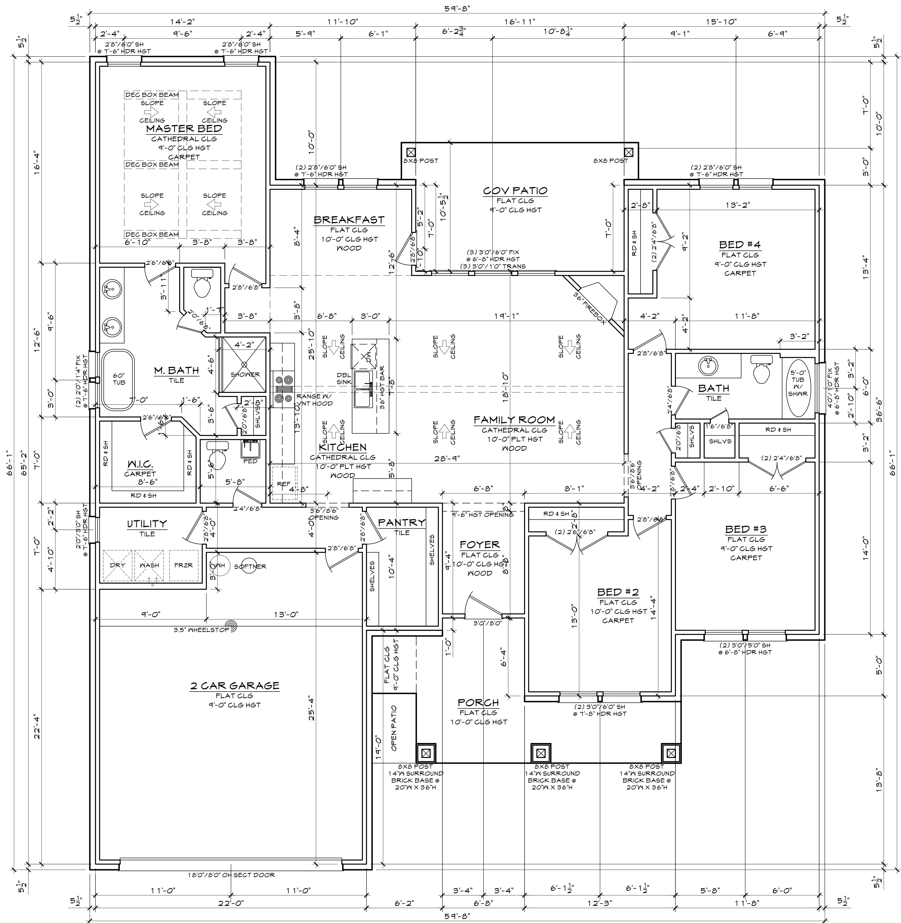
1 FLOOR PLAN A3 SCALE: 1/4" = 1'
