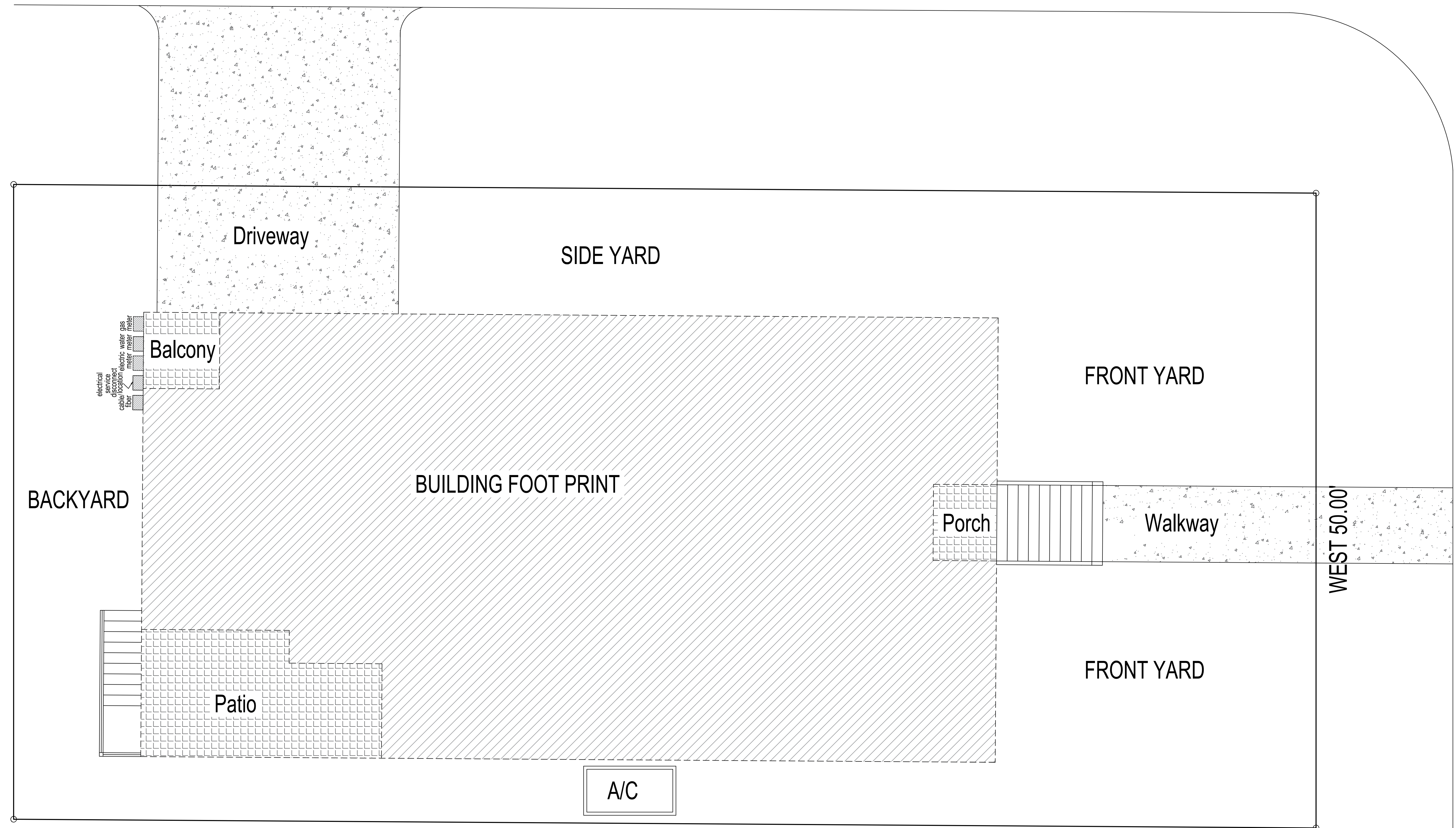
1 SITEPLAN
