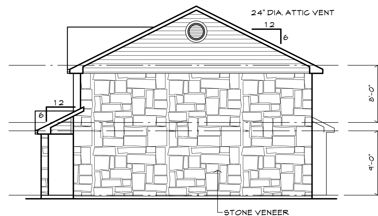
6 BLDG. E - RIGHT SIDE ELEV. 1/8" = 1'-0"
