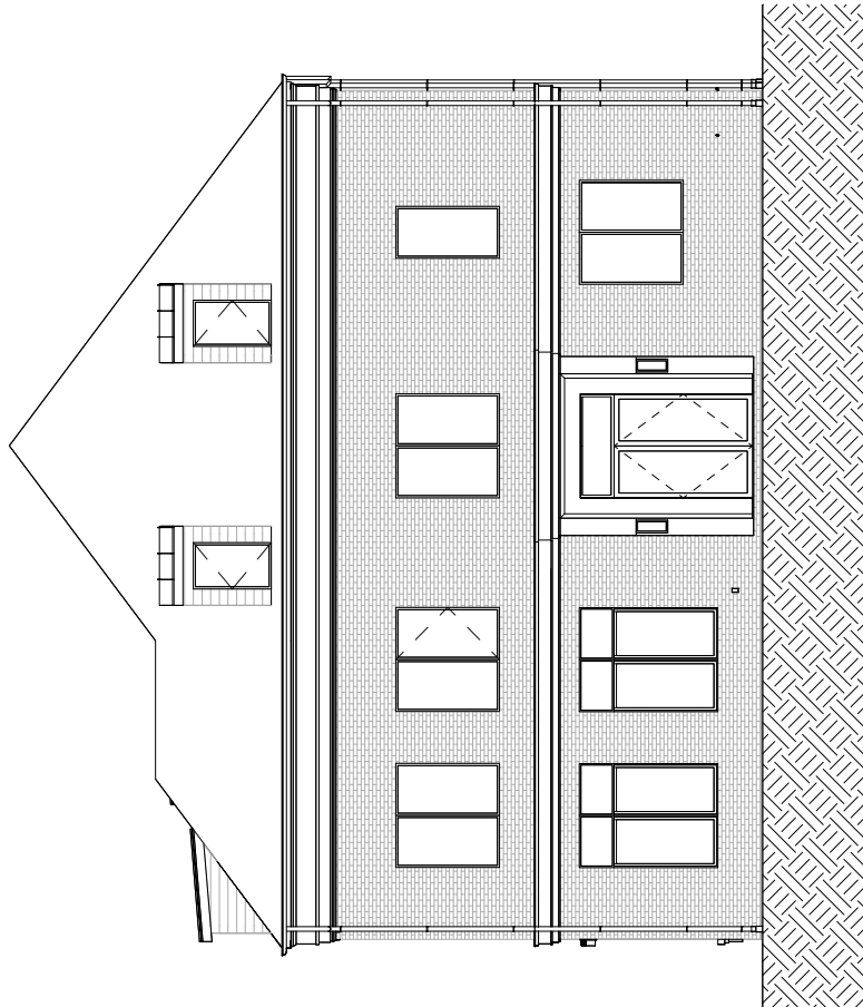
02 BACK ELEVATION GRAPHIC SCALE: 1/8" = 1'-0"
