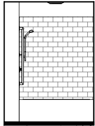
G. BATH ELEVATION - 2 | SCAL. 1/2" = 1'-0" | 10
