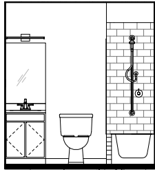
G. BATH ELEVATION - 1 | SCAL. 1/2" = 1'-0" | 9
