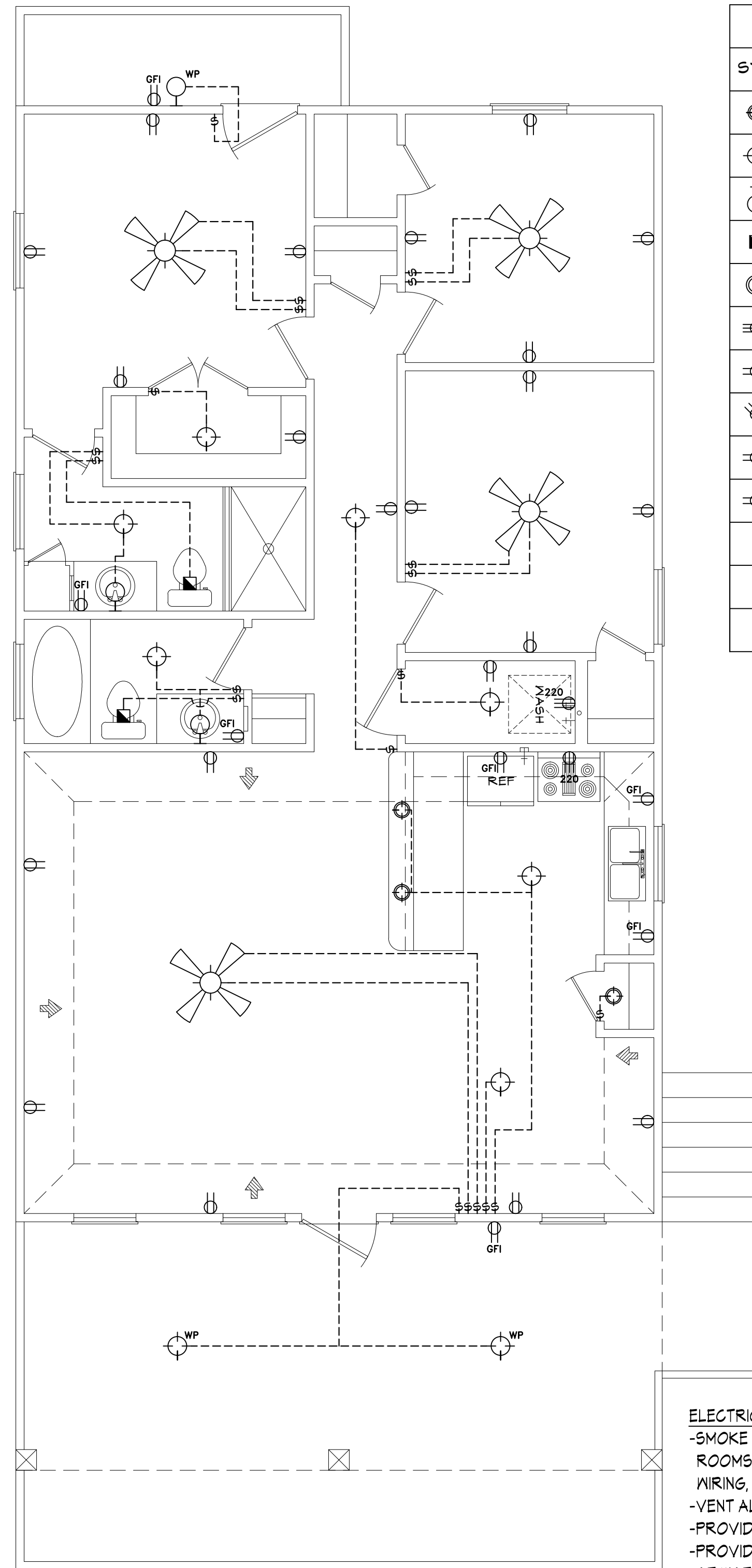
2 ELECTRICAL A3 SCALE: 1/4" = 1'
